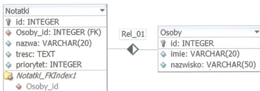
Ilustracja 1. Baza danych
