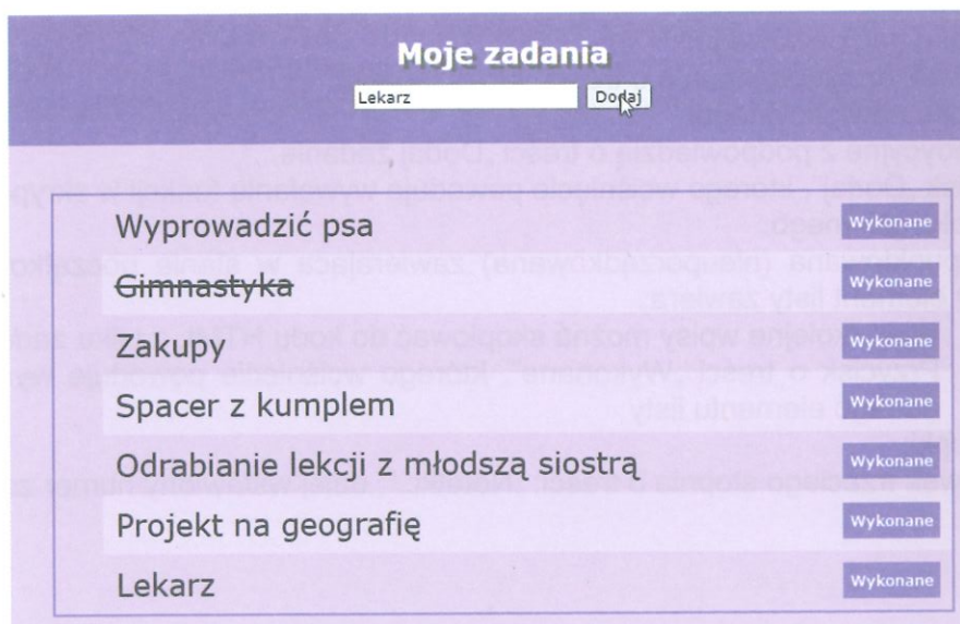
Ilustracja 4. Działanie aplikacji
